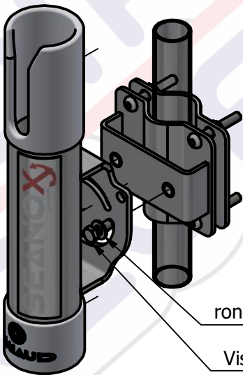
Exemple de montage bride simple avec porte canne ( porte canne non fourni)
